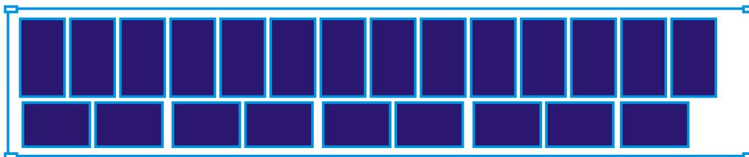
40-футов контейнер - 23 европалети (800 мм x 1200 мм) 40 foot container - 23 standard pallets (800 mm x 1200 mm)
