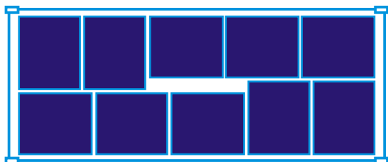
20-футов контейнер - 10 стандартни палети (1000 мм x 1200 мм) 20 foot container - 10 standard pallet (1000 mm x 1200 mm)
