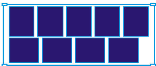
20-футов контейнер - 9 стандартни палети (1000 мм x 1200 мм) 20-foot container - 9 standard pallets (1000 mm x 1200 mm)
